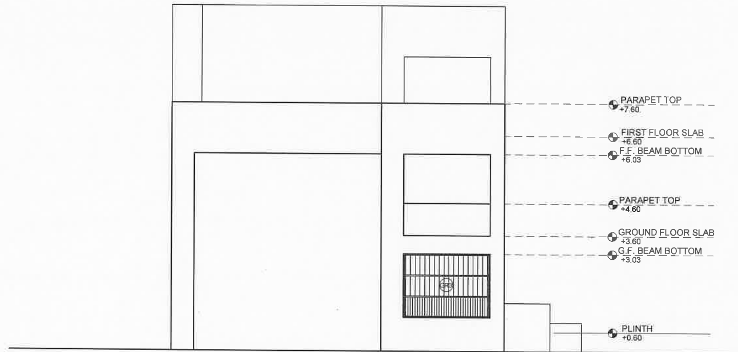
ELEVATION - B
