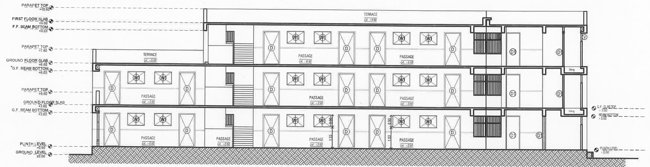
SECTION : 5-5
