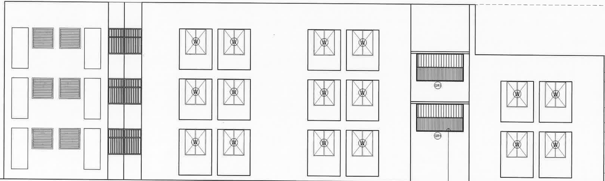
ELEVATION - C
